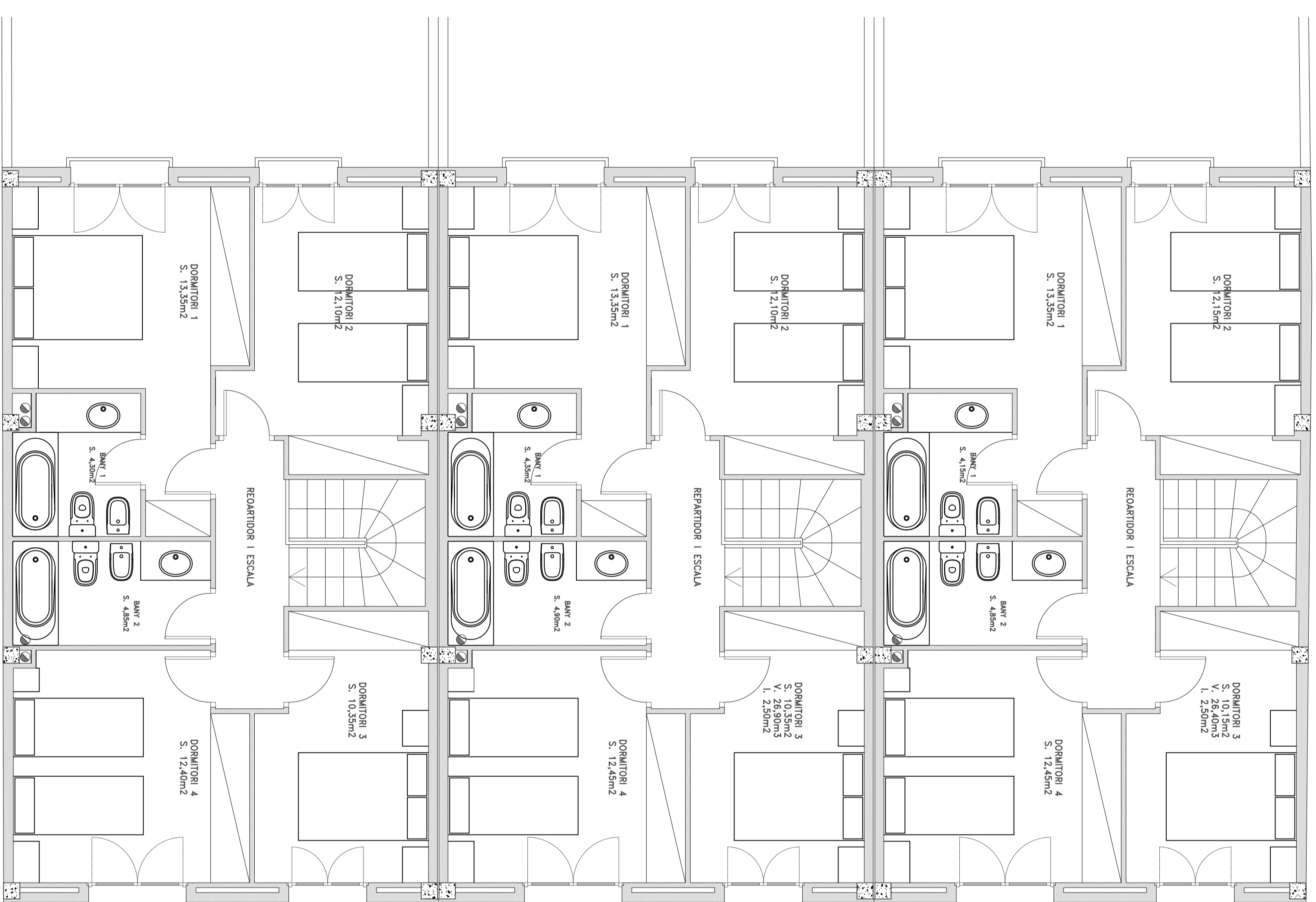
PLANTA PIS
