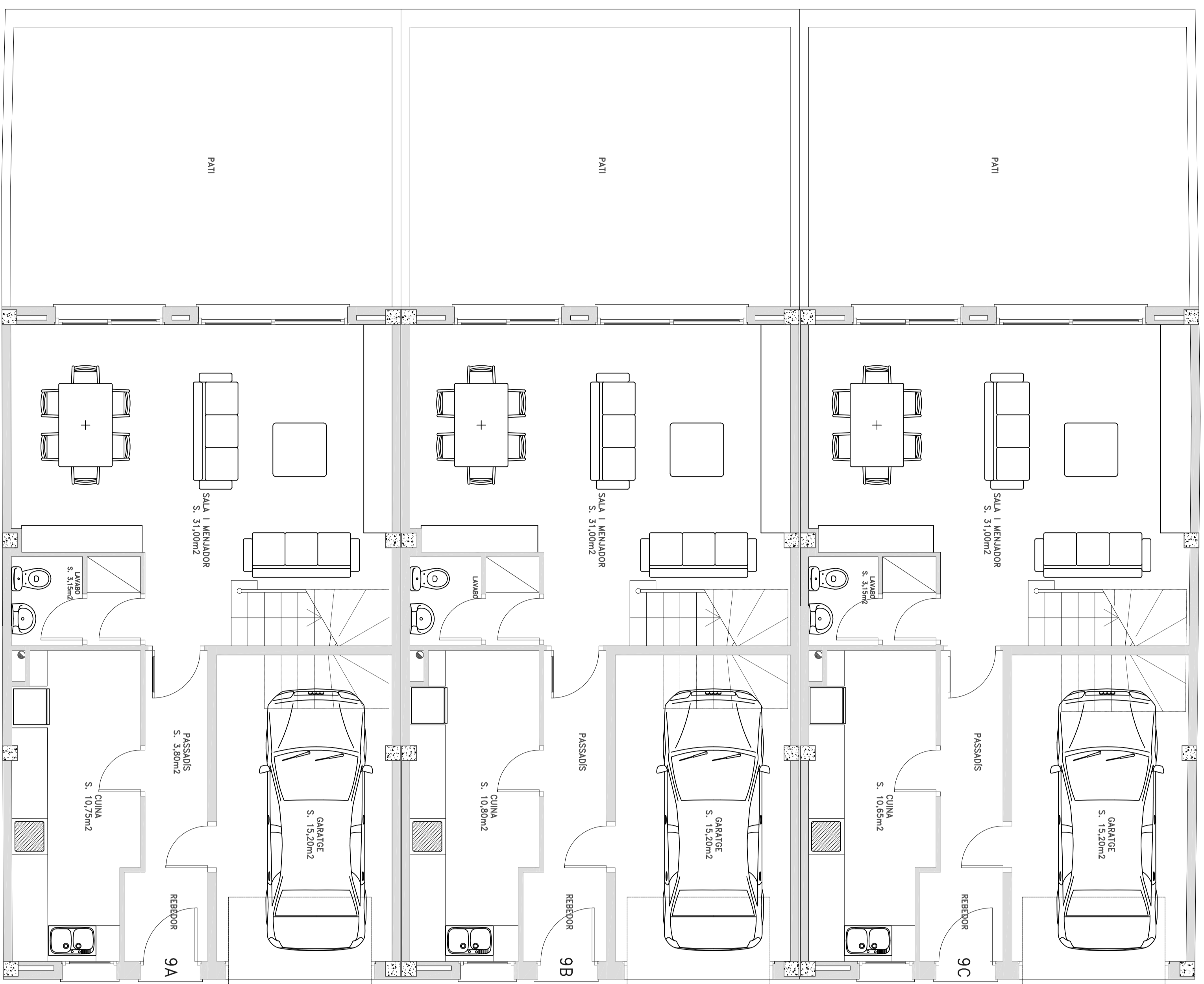
PLANTA BAIXA
